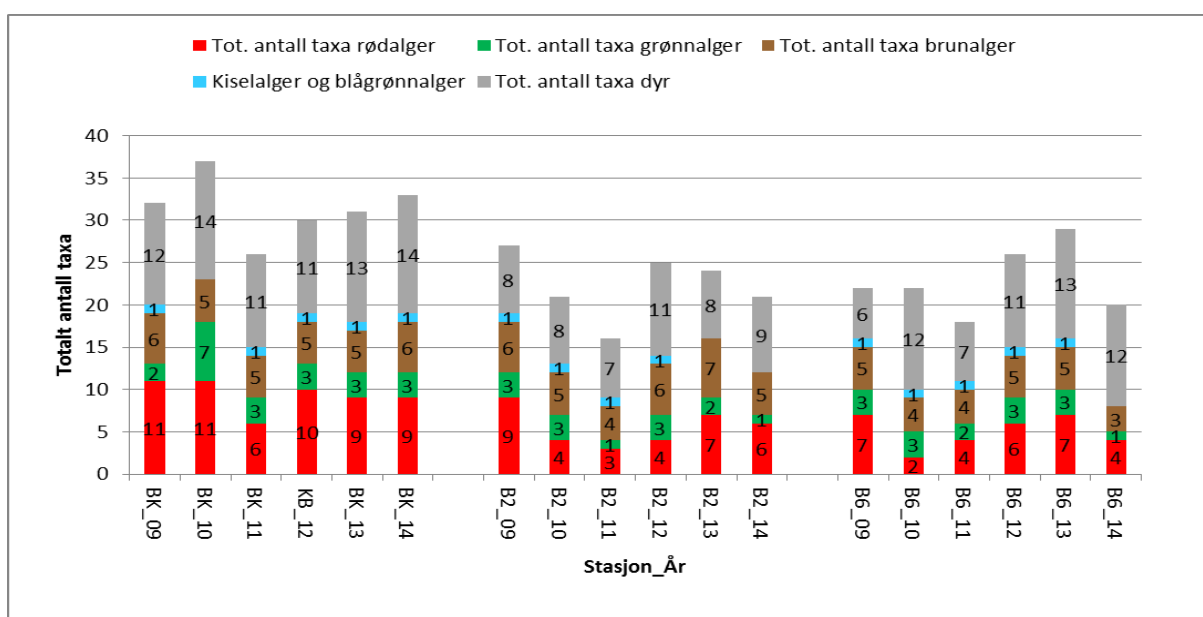
Figur 15. Antall taxa registrert på stasjonene BK, B2 og B6 i 2009 - 2014. Søylen viser totalt antall taxa registrert, fordelt på rødalger (rød), grønналger (grønn), brunalger (brun), kisel/blågrønnalger (blå) og dyr (grå).
