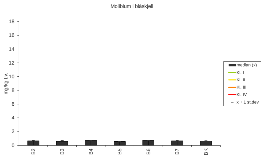
Figur 26. Median, standard avvik og nedre grense til Miljødirektoratet Klasse II og III konsentrasjon for molybden (ppm. (mg/kg tørrvekt) i blåskjell ( Mytilus edulis ) a. 2012, b. 2013 c. 2014.
