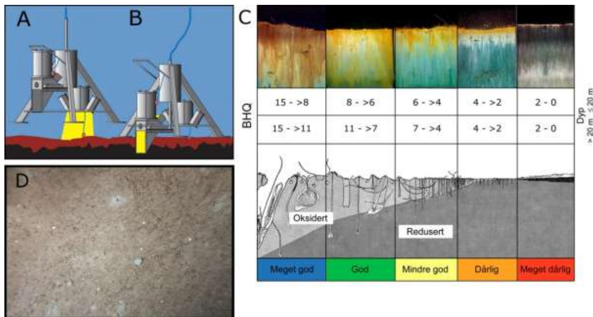
Figur 6. Prinsippskisse for SPI-kamera og bildeanalyse. (A) Rigg over bunnen. Gult antyder at bilde av overflaten tas. (B) Kamera med prismet som har trengt ned i sedimentet og SPI bildet eksponeres. (C) Figuren viser en modell av endringer i faunatype fra upåvirkede bunnsedimenter med en rik, dyptgravende fauna (Meget god) til en grunnlevende, fattig fauna i påvirkede områder (Meget dårlig). Sedimentprofilbildet er vist i toppen av figuren, der brunt farget sediment indikerer oksidert, bioturbert sediment mens sortfarget sediment indikerer reduserte forhold. Grenseverdier for BHQ-miljøkvalitetsindeks for vanddyb \leq 20 meter og > 20 m i samme skala som benyttes for marine sedimenter i EUs vanndirektiv (Pearson & Rosenberg 1978, Nilsson & Rosenberg 1997, Rosenberg et al. 2004, Nilsson & Rosenberg 2006 er vist). (D) Eksempel av et overflatebilde med strukturer og børstemarkrør synlig.
